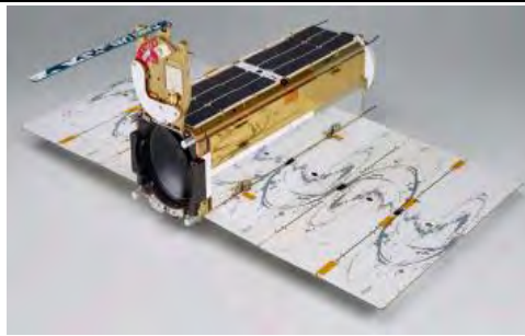
※小型の CubeSat 衛星「Dove」の外形寸法は 10x10x30cm、重量は 4~5kg。
