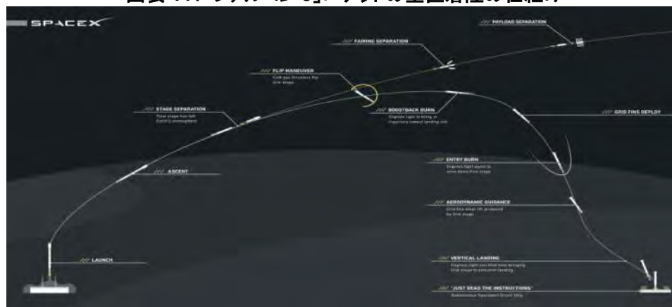
図表 11:「ファルコン 9」ロケットの垂直着陸の仕組み
